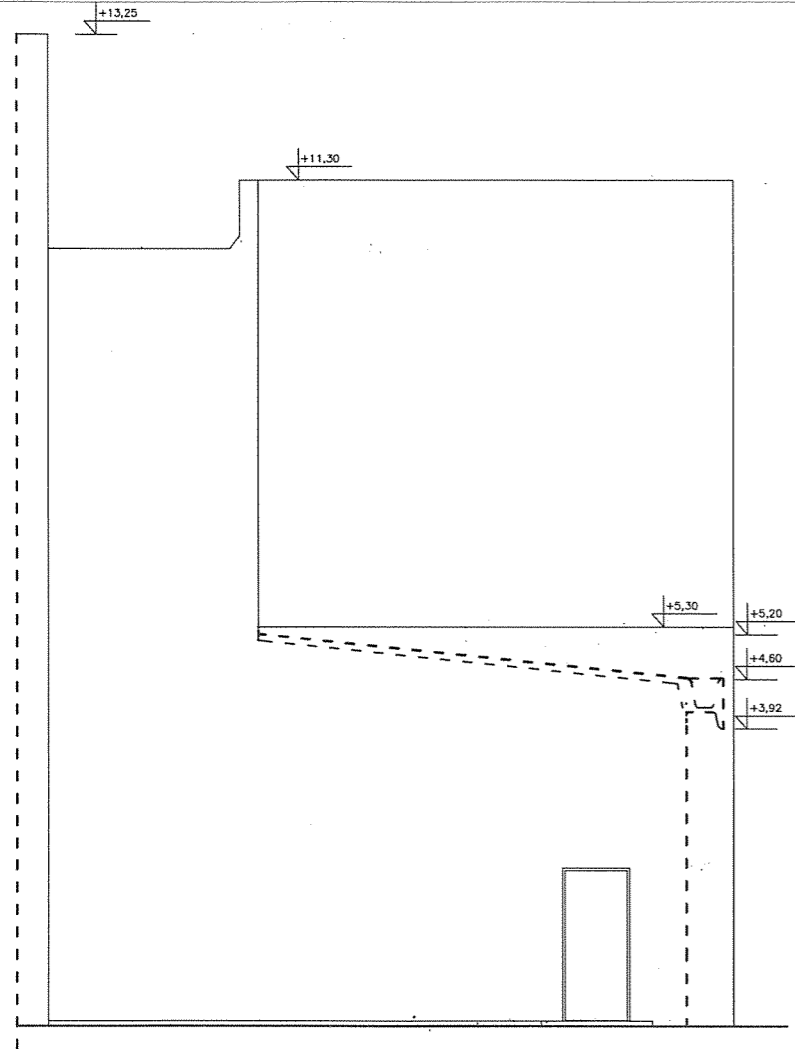
ELEWACJA-STAN ISTN. 1:50
