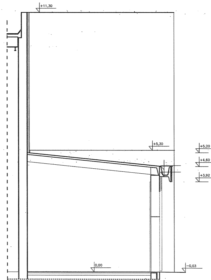
PRZEKRÓJ-STAN PROJ. 1:50
