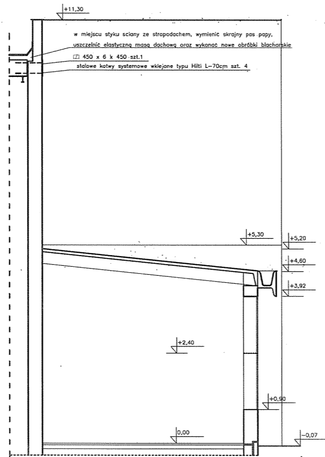
PRZEKRÓJ-STAN ISTN. 1:50
