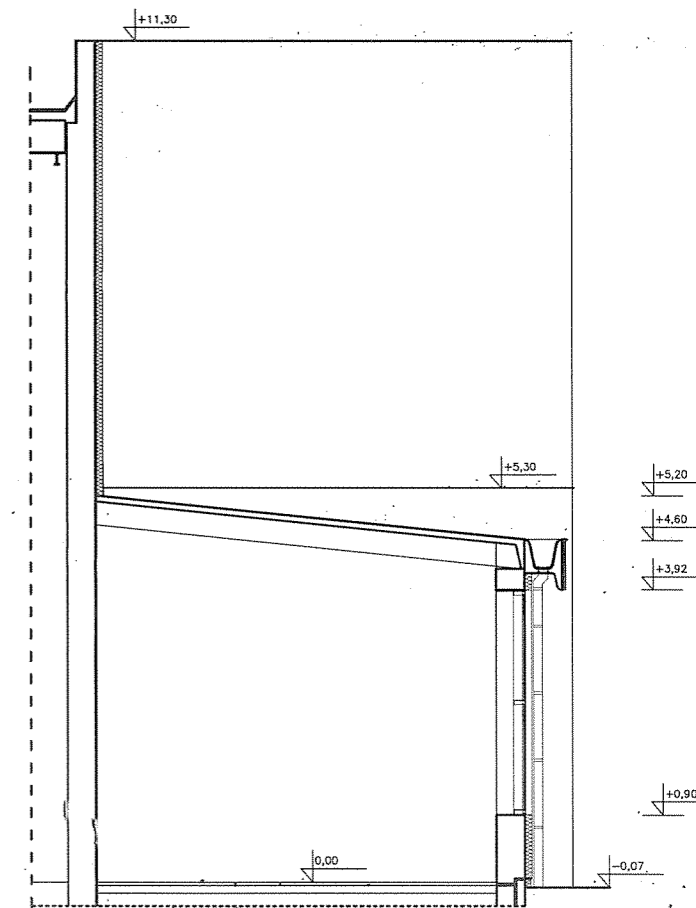
PRZEKRÓJ - STAN PROJ. 1:50
